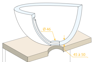
▶ AVEC TROP-PLEIN INTÉGRÉ.
