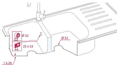
Ø 50 SIMPLE PAROI : inox.
