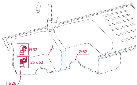
Ø 60 SIMPLE PAROI : synthèse, céramique.
