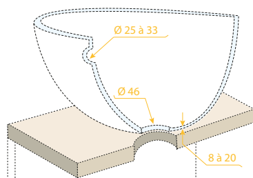
▶ AVEC TROP-PLEIN EXTÉRIEUR.
