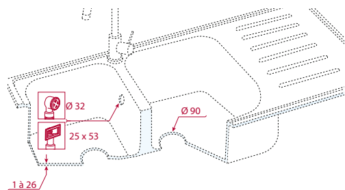
Ø 90 SIMPLE PAROI : inox, synthèse, céramique.
